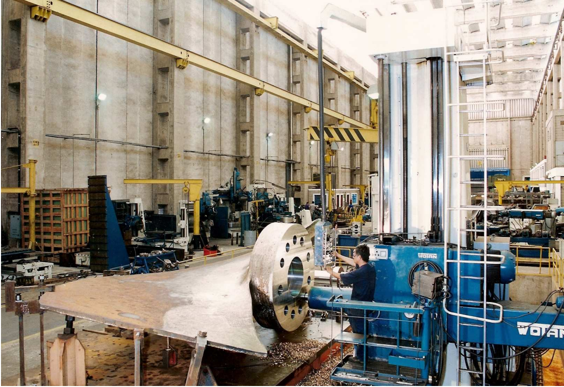
Foto 4 - Vista parcial do parque fabril - Mandriladora Wotan.
