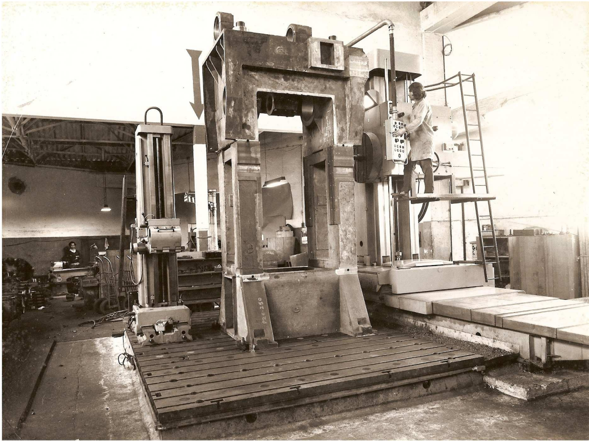
Foto 5 - Operação de usinagem no corpo de uma prensa de duas colunas.
