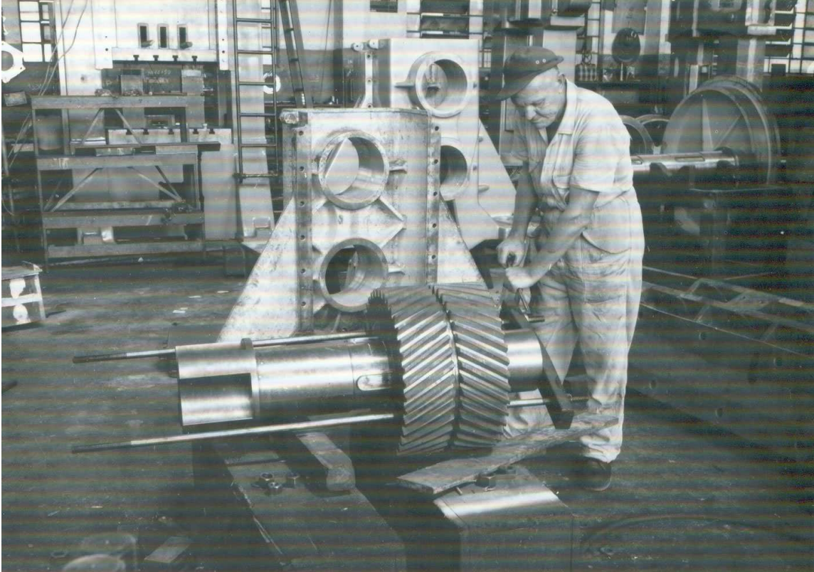
Foto 6 - Profissional ajustando conjunto de pinhão bi-helicoidal.
