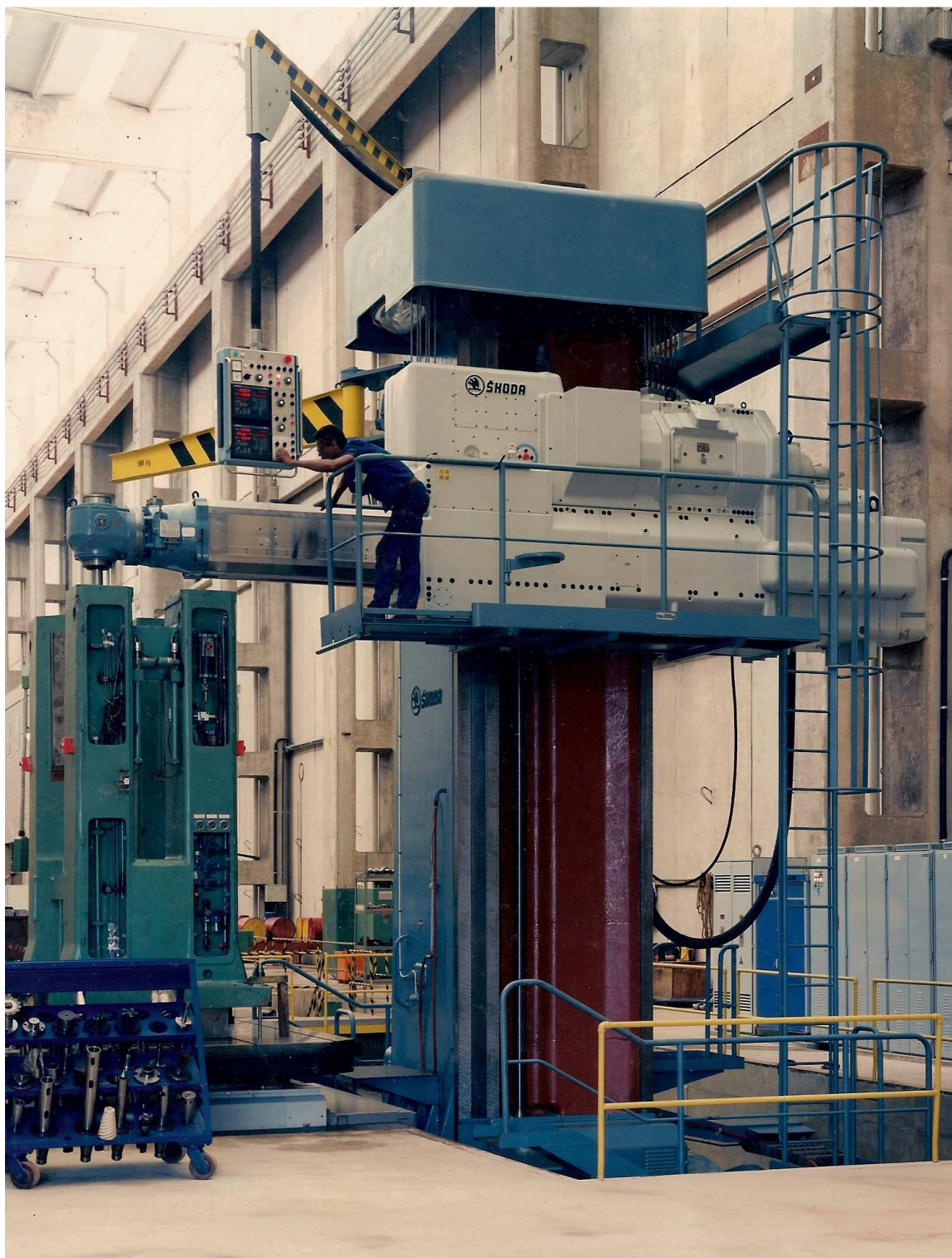
Foto 7 - Vista parcial do parque fabril - Mandriladora Skoda.
